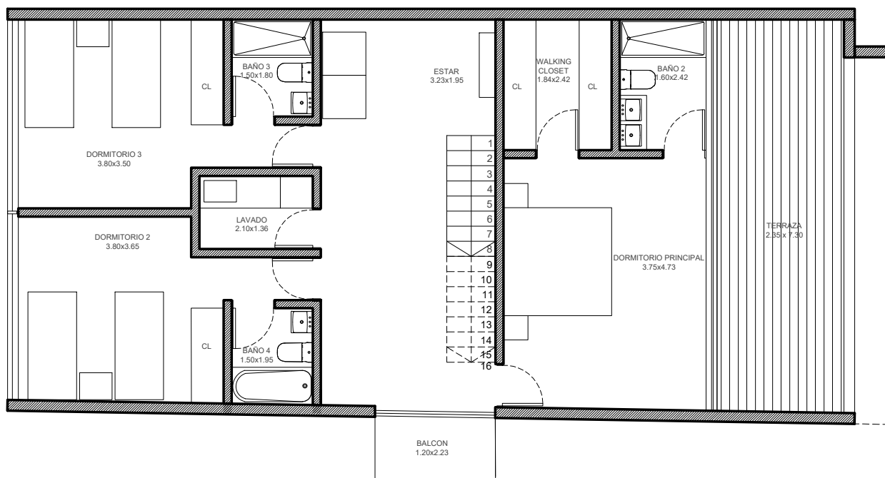
PLANTA SEGUNDO PISO
